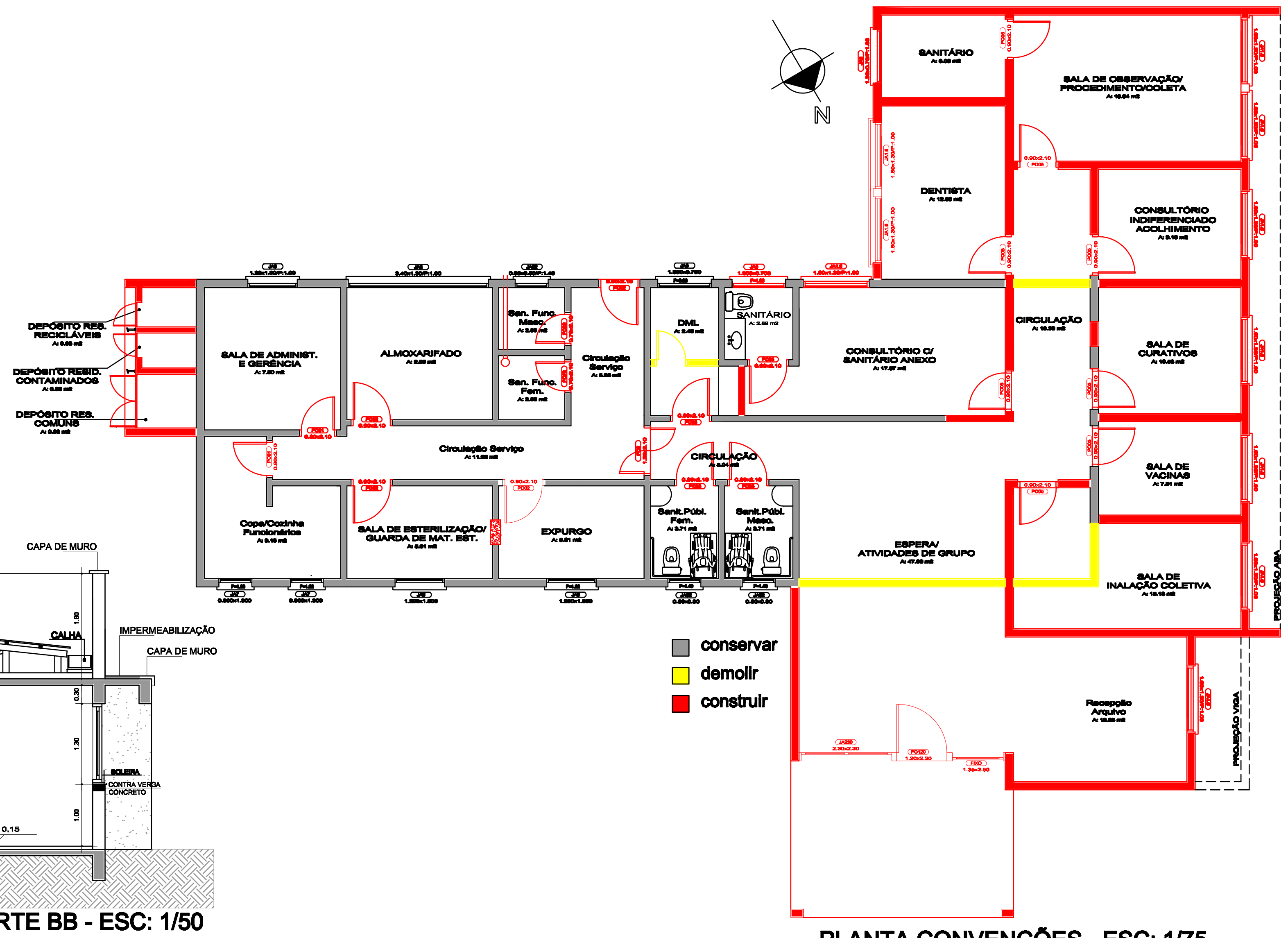
PLANTA CONVENÇÕES - ESC: 1/75
