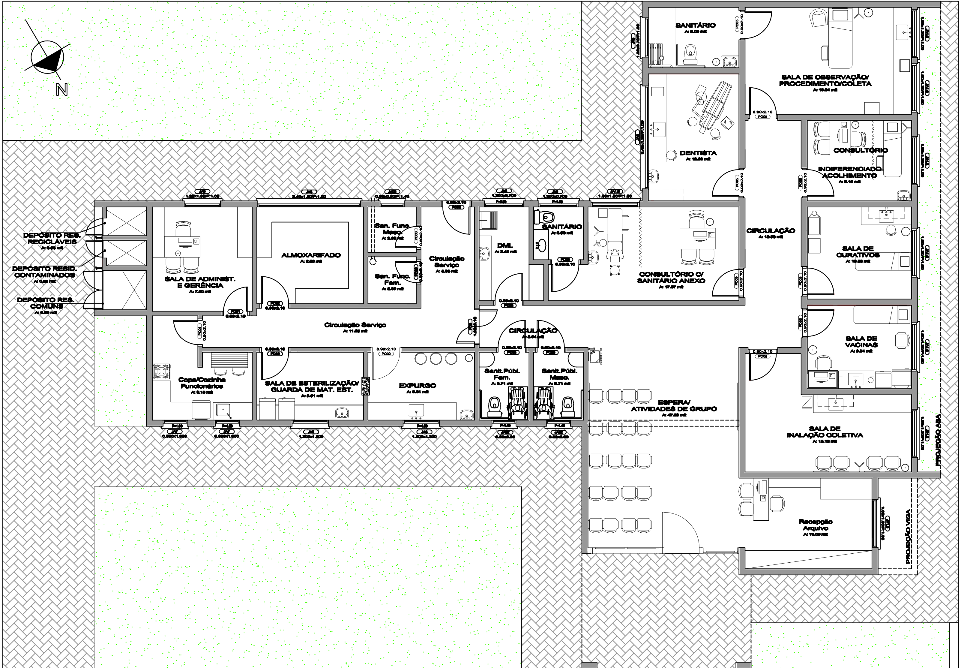
PLANTA LAY DE OUT - ESC: 1/75
