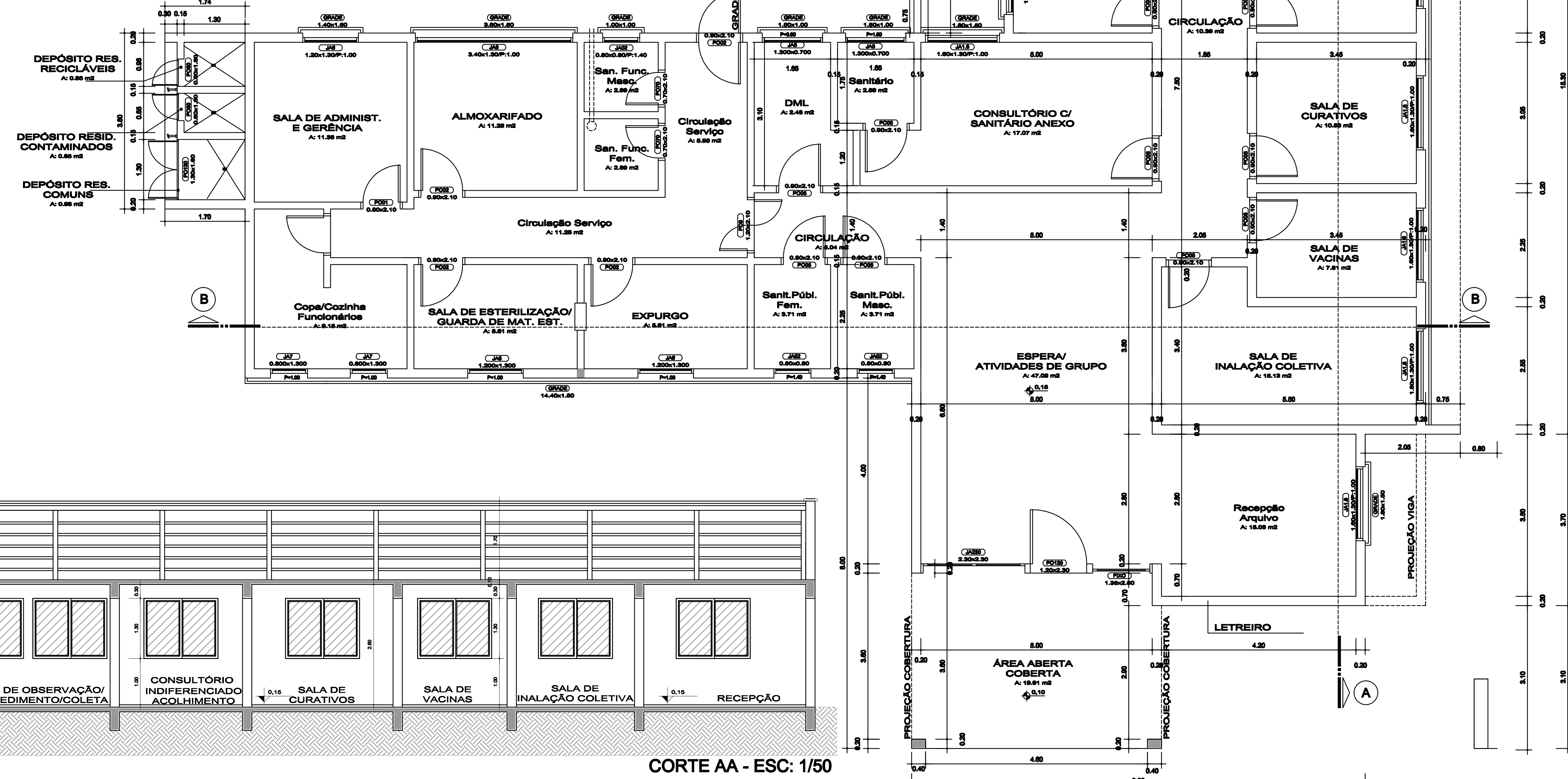
PLANTA BAIXA COTADA - ESC: 1/50
